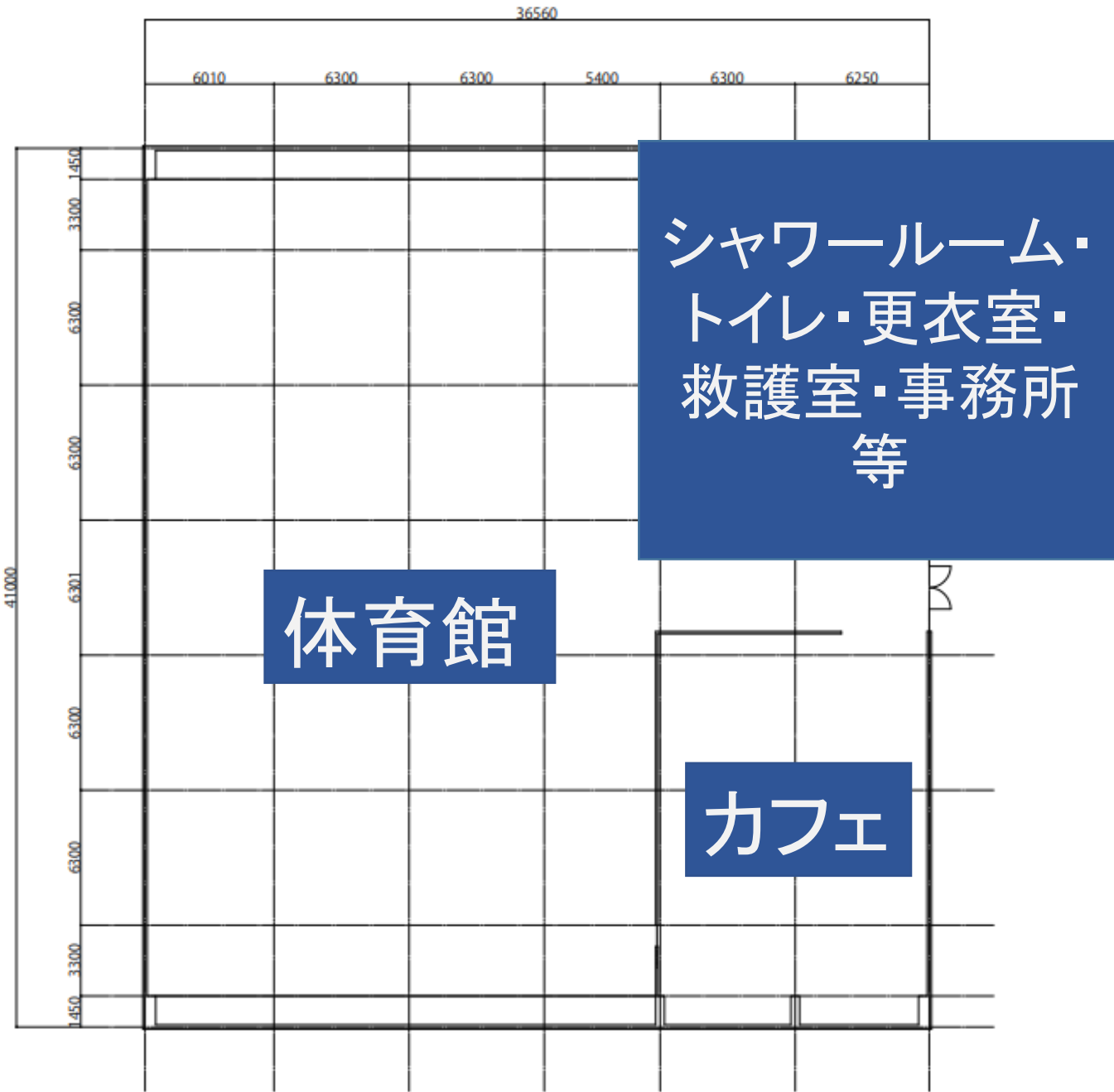
1:200 体育館 平面図
